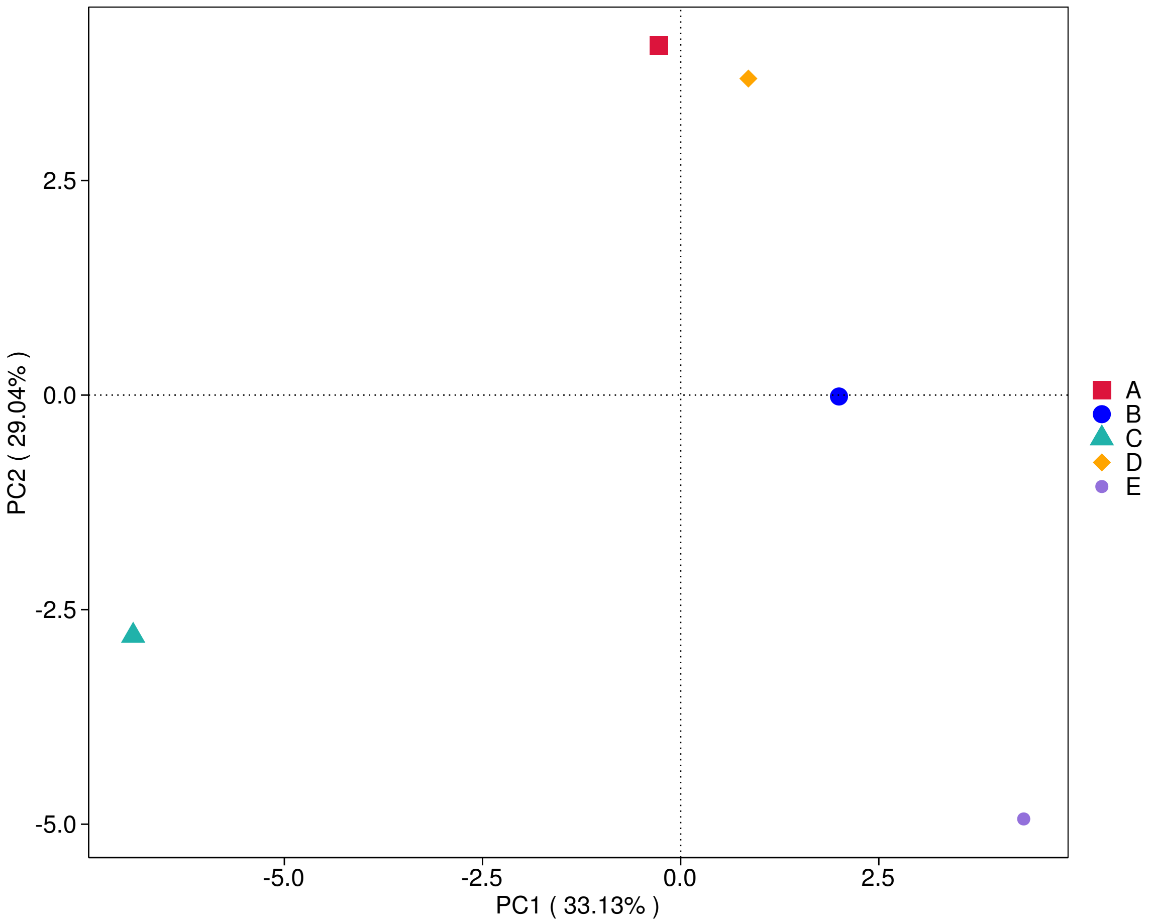
PCA Plot
