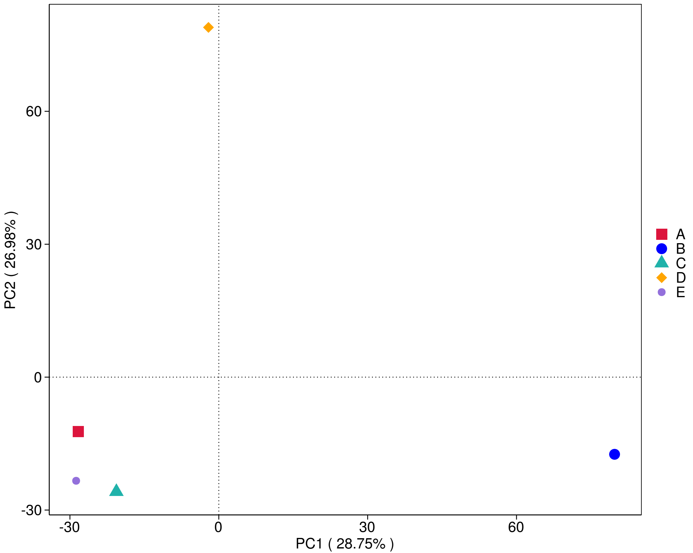
PCA Plot
